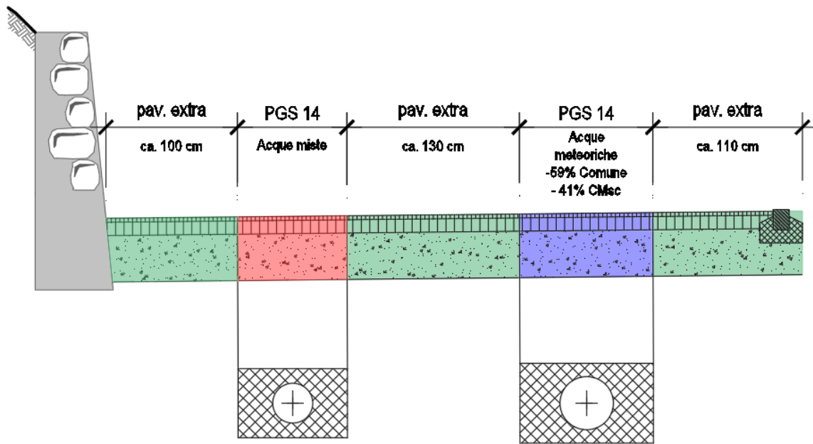
Figura 1: sezione tipo pavimentazione strada cantonale
